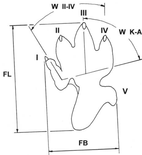
Abb. 3: Wichtige Messgrößen am vorliegenden Trittsiegel von Chirotherium barthii . FL = Länge des Fußeindrucks, FB = Breite des Fußeindrucks, W II-IV = Winkel zwischen den Zehen II – IV, W K-A = Winkel der Kreuzachse: Verbindung der Metatarsus-Phalangen-Gelenke I und IV zur Mittelachse von Zehe III.
