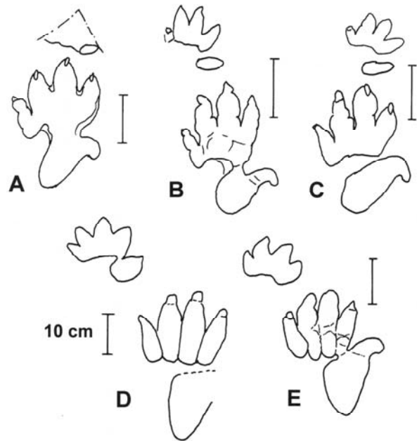
Abb. 4: Vergleich des beschriebenen Trittsiegels von Chirotherium barthii (A) mit zwei Ausprägungen von Chirotherium barthii (B, C) und Chirotherium rex (D) sowie „ Chirotherium moquinense “ (E) aus der Moenkopi-Formation Nordamerikas. B – E nach PEABODY aus KLEIN & LUCAS 2010.
